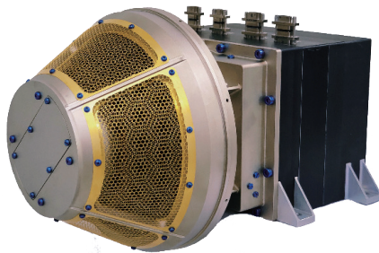
Fig. 8 FM of LIA
