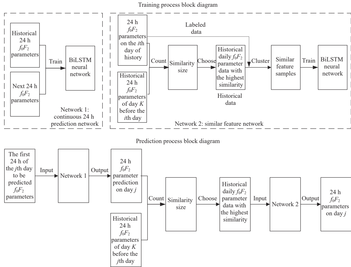
图 3 基于电离层参数相似特征的深度学习预测模型的训练及预测流程
