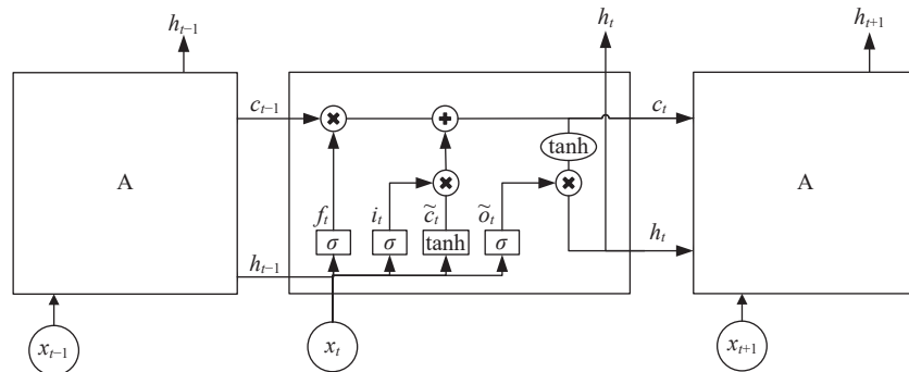
图 1 LSTM 神经网络结构 Fig. 1 LSTM neural network structure diagram
