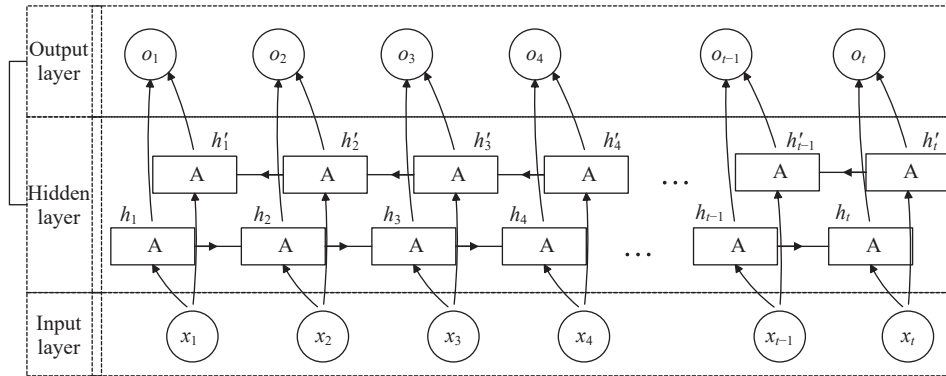
图2 BiLSTM神经网络结构
