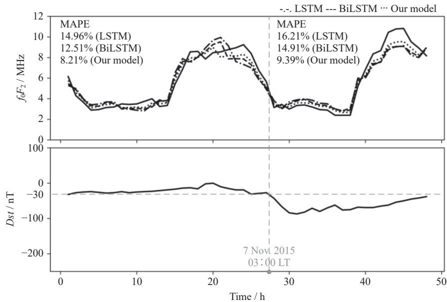
图6 2015年11月6日00:00 LT至2015年11月7日23:00 LT地磁暴期间 f_0F_2 参数预测结果
