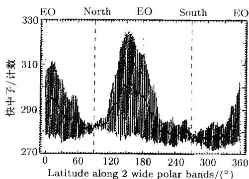
图 3 LP 快中子探测结果剖面图
