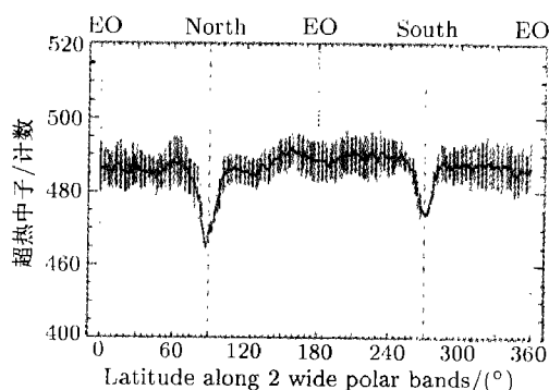
图 2 LP 超热中子探测结果剖面图
