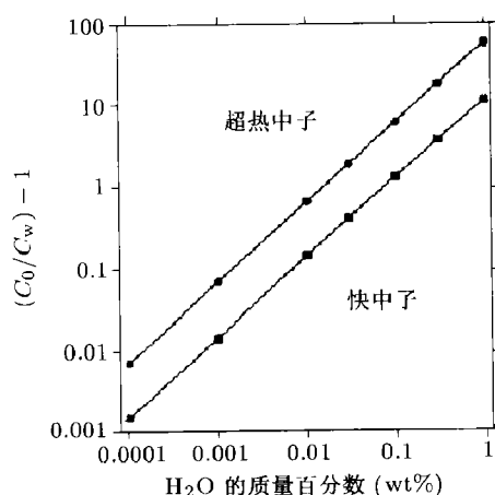
图 4 FAN(铁质钙长石质) 月壤中超热中子和快中子记数率与水含量之间的关系 ( C 为计数率)
