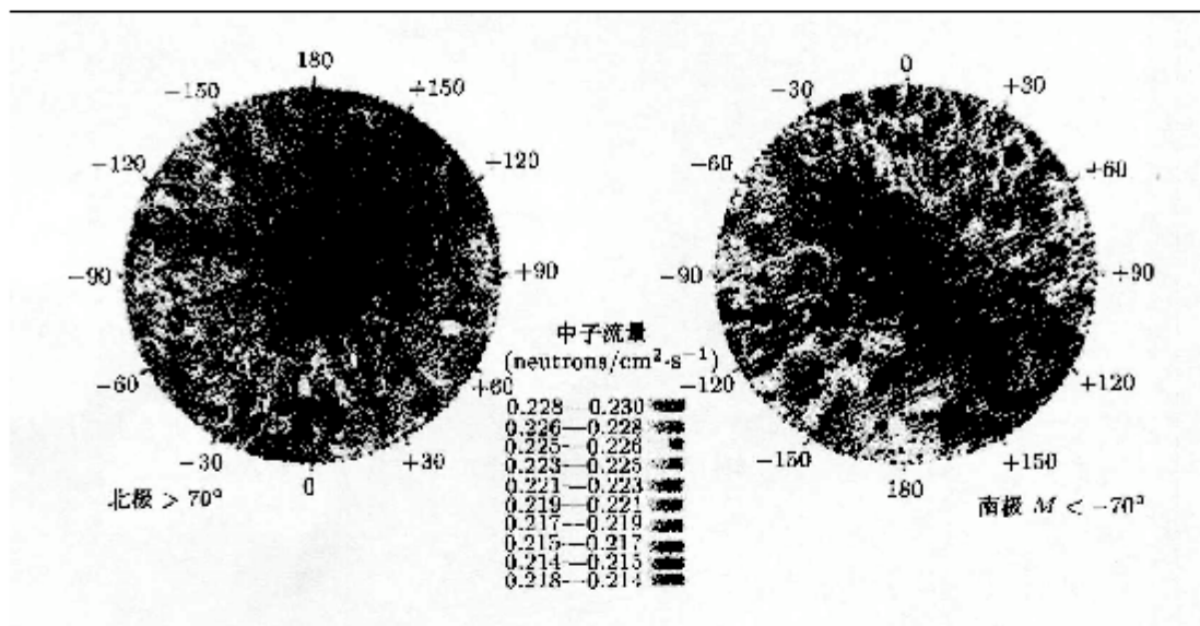
图 1 月球极区的超热中子计数率图
