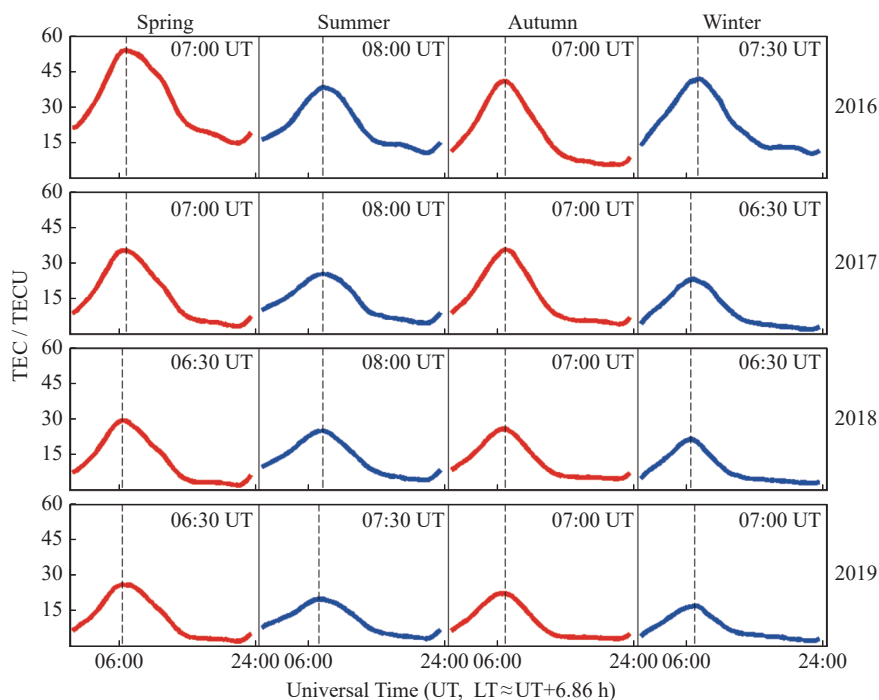
图 2 TEC 在 2016—2019 年季节平均的日变化 (虚线为各季节平均最高值对应的时间)
