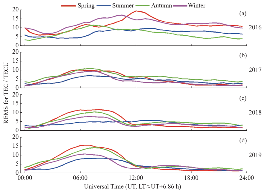
图5 IRI-2020 对观测值的均方根偏差值在不同季节的变化
