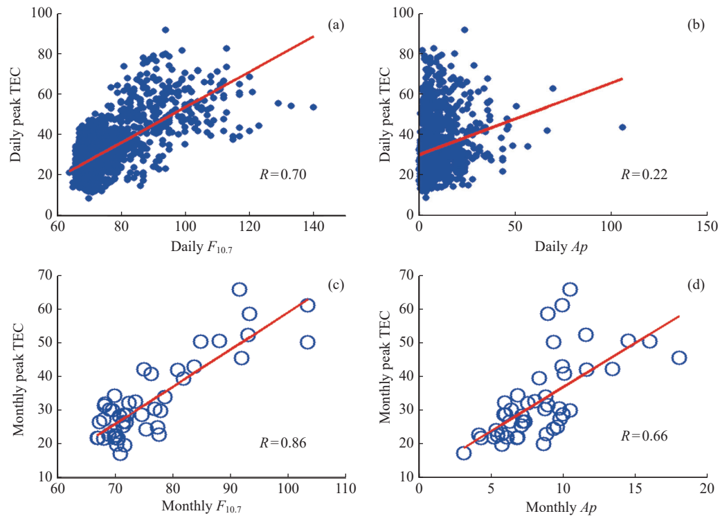
图3 TEC日最大值和月均最大值与 F_{10.7} 及 A_p 指数之间的相关系数 ( R 为线性相关系数,红色直线是线性拟合结果)
