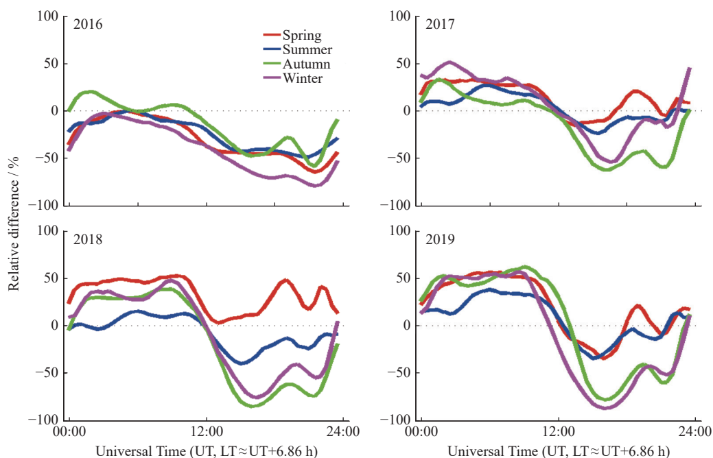
图 6 IRI-2020 对观测值的相对偏差在 2016—2019 年中随季节和时间的分布
