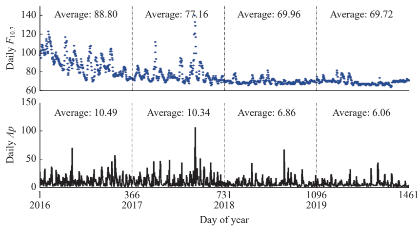
图 1 2016—2019 年 F_{10.7} 及 A_p 指数的变化情况
