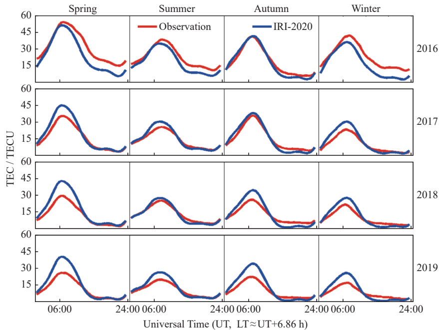
图 4 TEC 观测值与 IRI-2020 模拟的季节平均值对比
