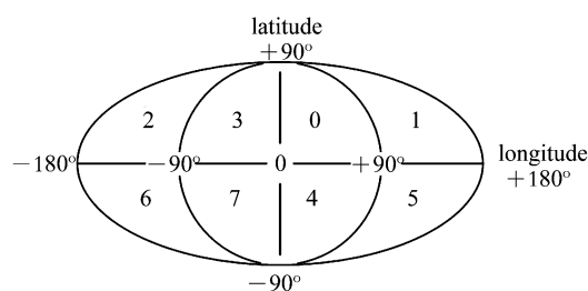
图 6 八分体编码
