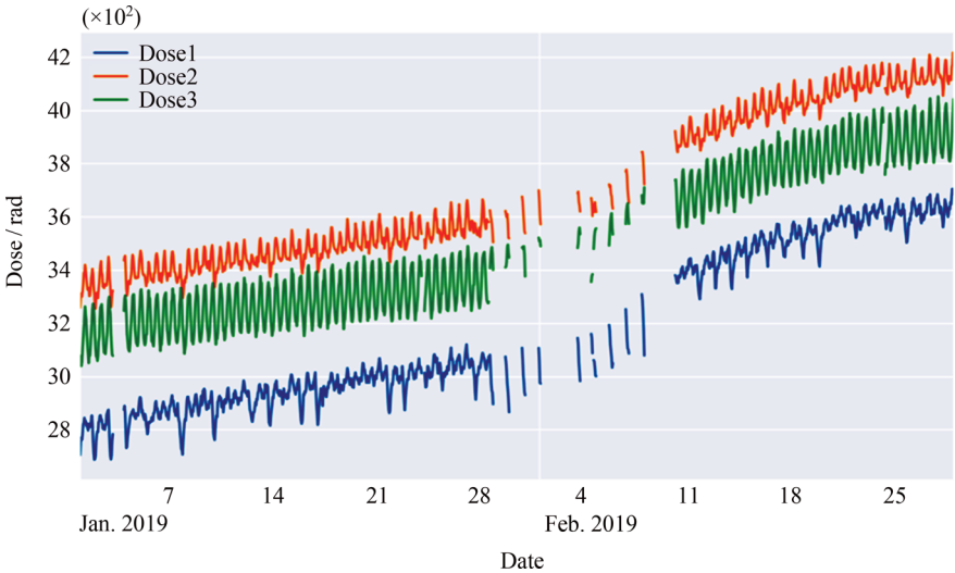
图2 2019年1月1日至2月28日卫星舱内三个方向辐射剂量变化曲线 Fig.2 Radiation dose curve in three directions in satellite cabin from 1 January to 28 February in 2019
