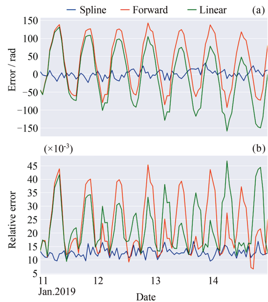
图 7 三种方法填充值与真实值误差 (a) 及相对误差 (b) 的对比情况 Fig. 7 Comparison of the error (a) and relative error (b) between filled values and real values of three methods
