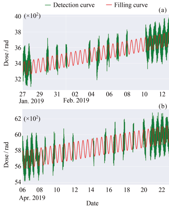
图 5 2019 年 1 月 27 日至 2 月 13 日和 4 月 6 日至 4 月 23 日辐射剂量变化曲线
