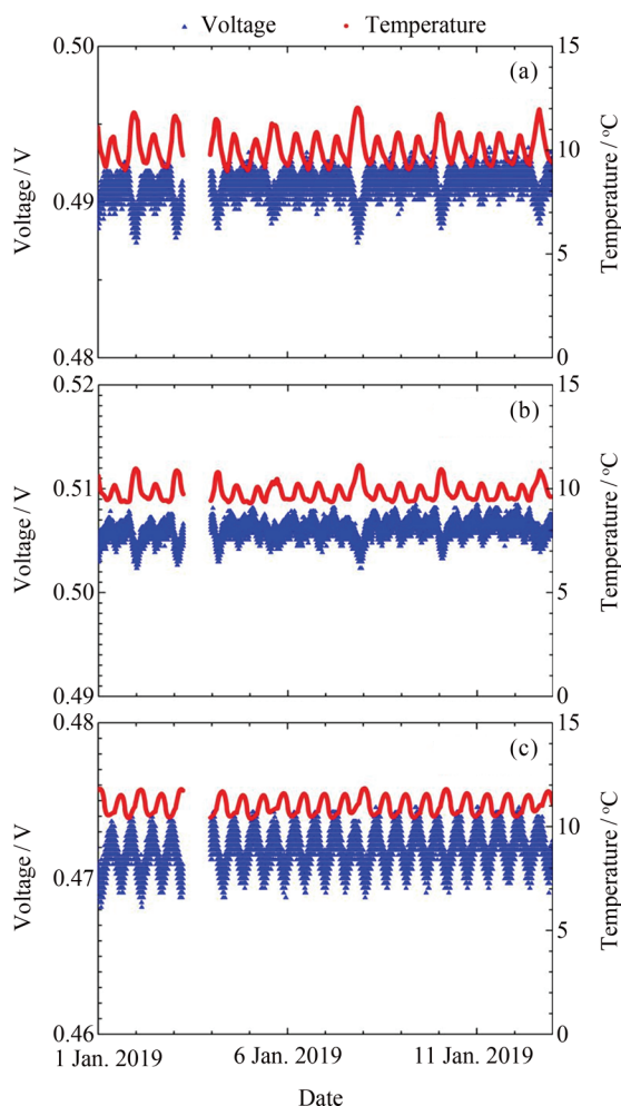
图 3 卫星舱内三个方向辐射剂量探测仪传感器输出电压与仪器温度的变化
