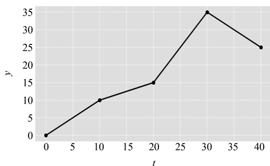
图 4 线性样条
