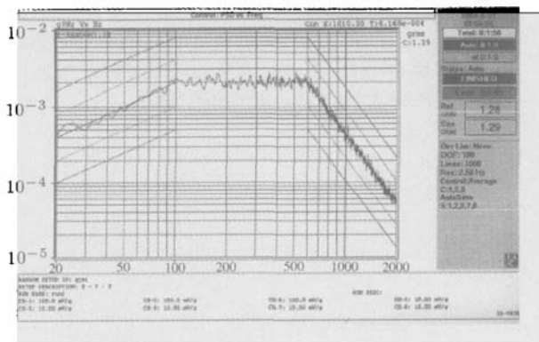
图 4 功率谱密度曲线 Fig.4 Power spectrum density curve
