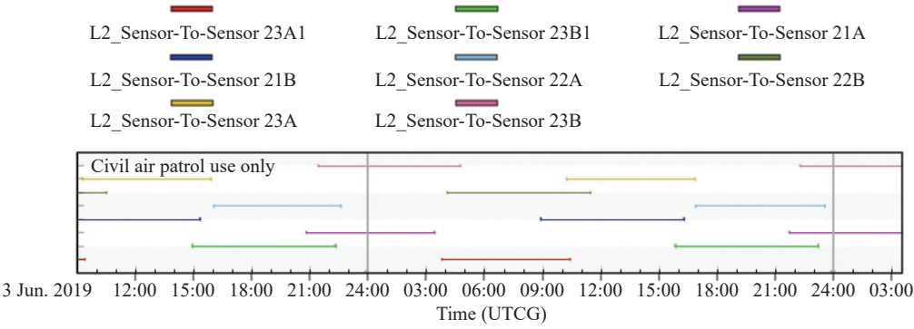
图 7 加装天地载荷的四节点天链星覆盖仿真
