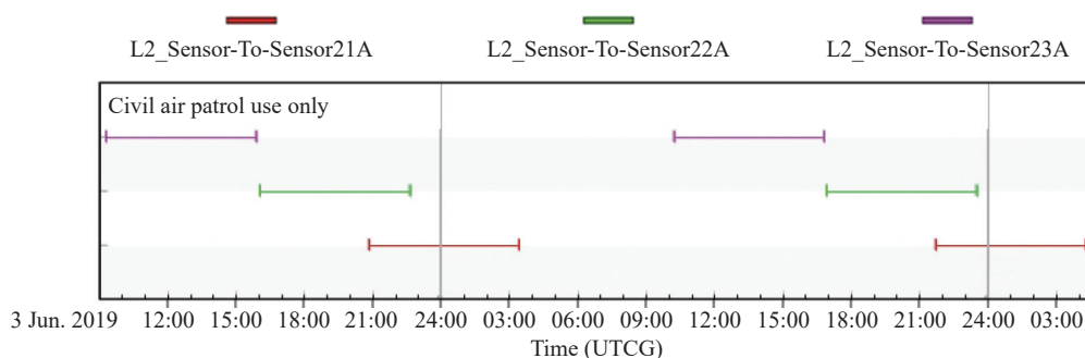
图3 当前天链星覆盖仿真
