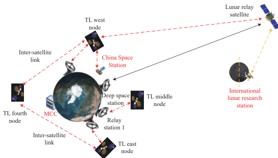
图 11 国际月球科研站通信链路
