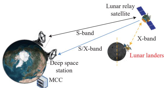
图1 嫦娥四号单星中继通信链路
