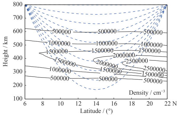
图1 模拟电离层背景场电子密度分布(虚线为模拟掩星射线路径)
