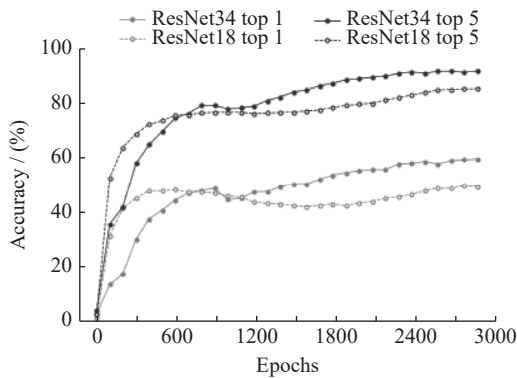
图 6 不同编码器结构的 MoCo 表征学习的准确率变化曲线
