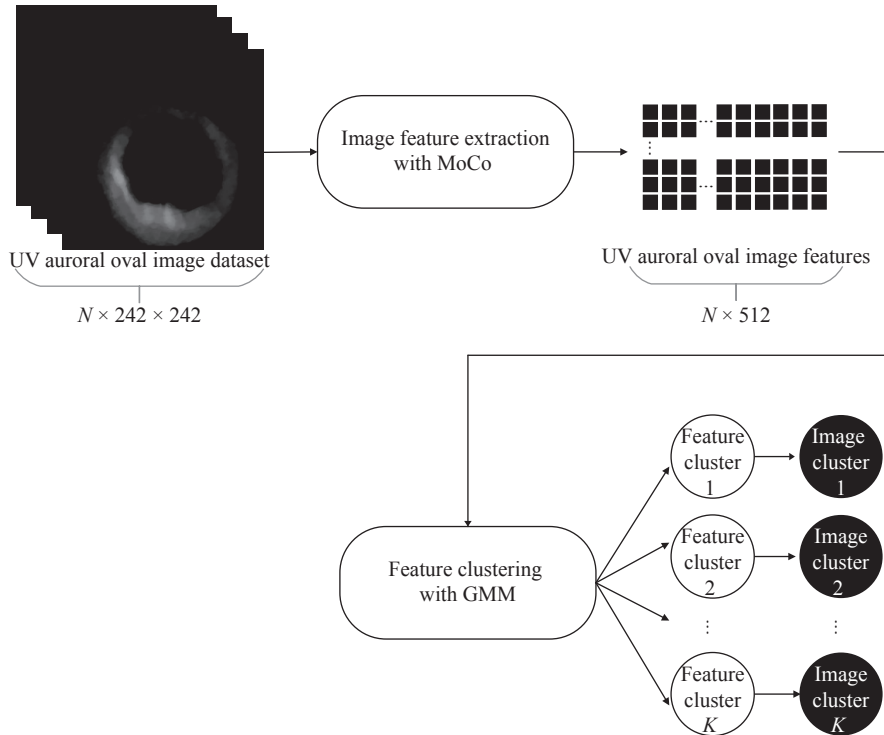
图 1 紫外极光卵图像聚类流程
