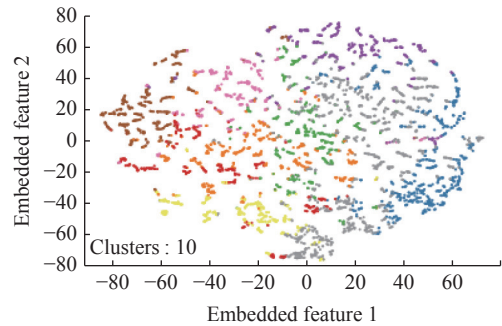
图 8 GMM 10-聚类结果可视化
