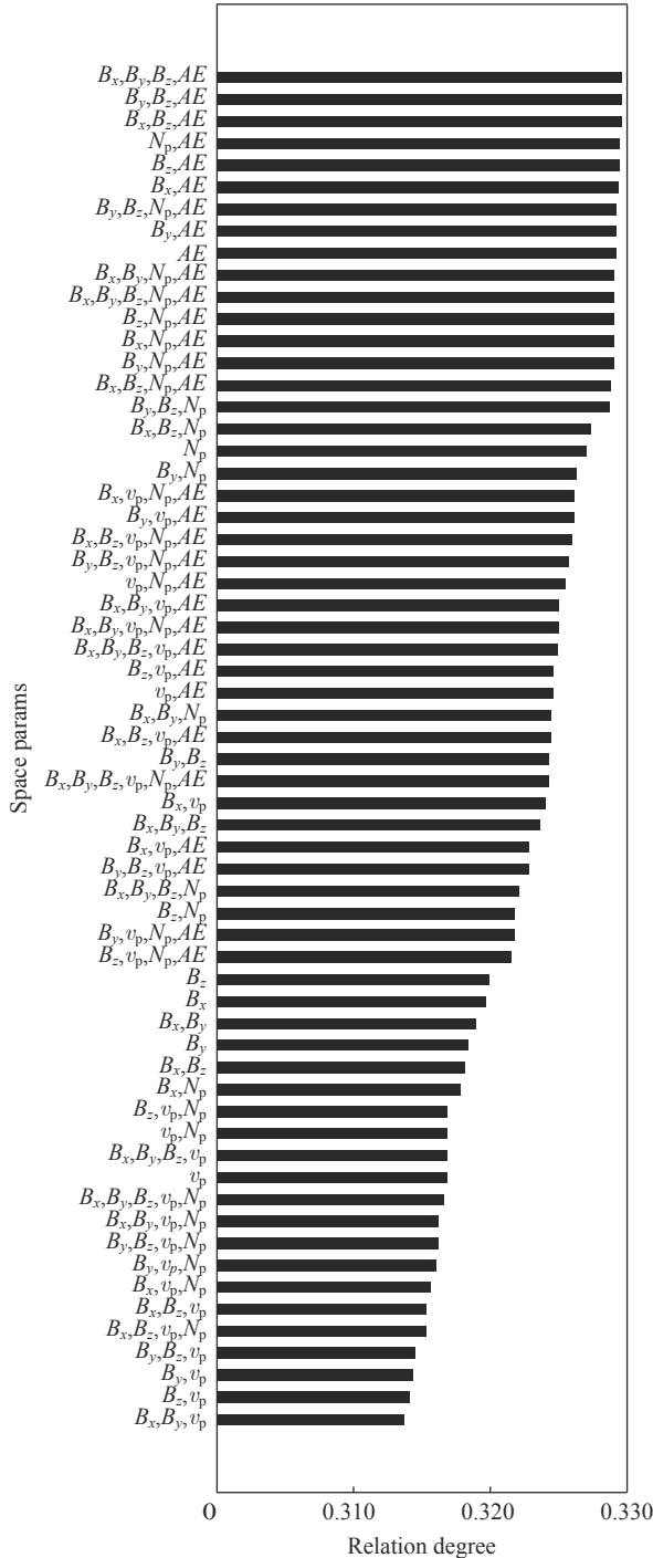
图 11 不同空间环境参数组合与紫外极光卵图像 10-聚类结果的关联度
