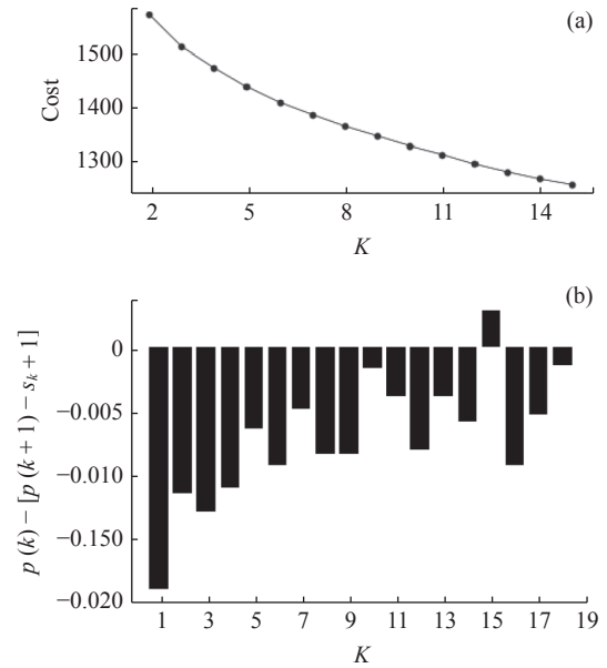
图 7 预估聚类簇数 K 。(a) Cost- K 曲线, (b) 间隔统计量法条状图
