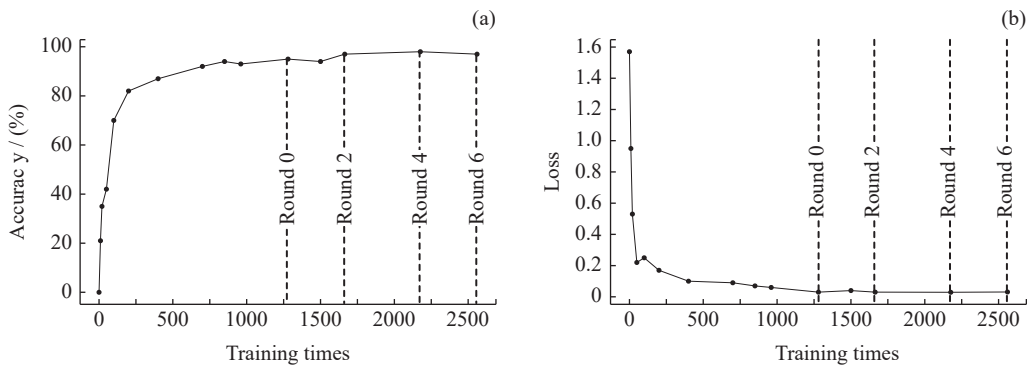
图 3 VggNet-16 迭代式分类的准确率和损失值变化曲线
