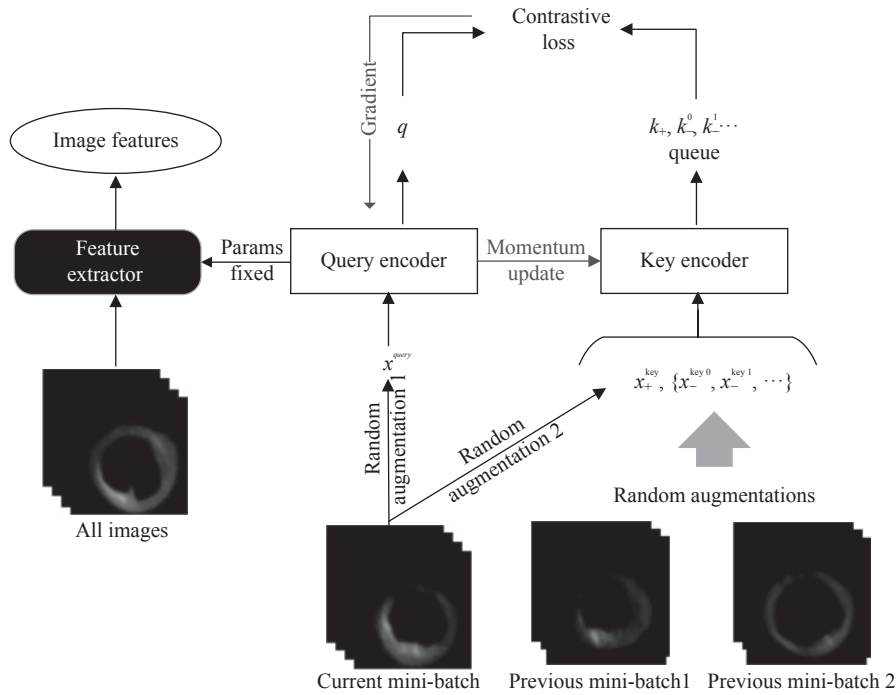
图2 MoCo 对比学习紫外极光卵图像表征
