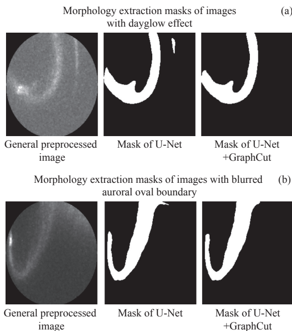
图 4 不同模型对日晖干扰图像和极光卵边界模糊图像的形态提取掩膜对比
