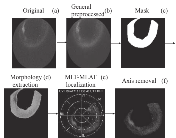
图 5 紫外极光卵图像数据预处理管线及效果
