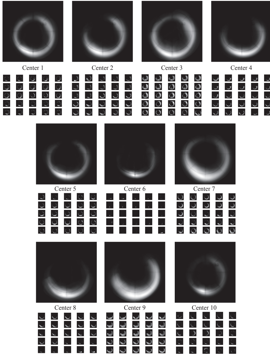
图9 POLAR 紫外极光卵图像 MoCo-GMM 10-聚类结果
