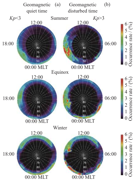
图 2 2018 年 3 月至 2019 年 11 月不同季节 JME 雷达在地磁平静期和扰动期的回波发生率分布
