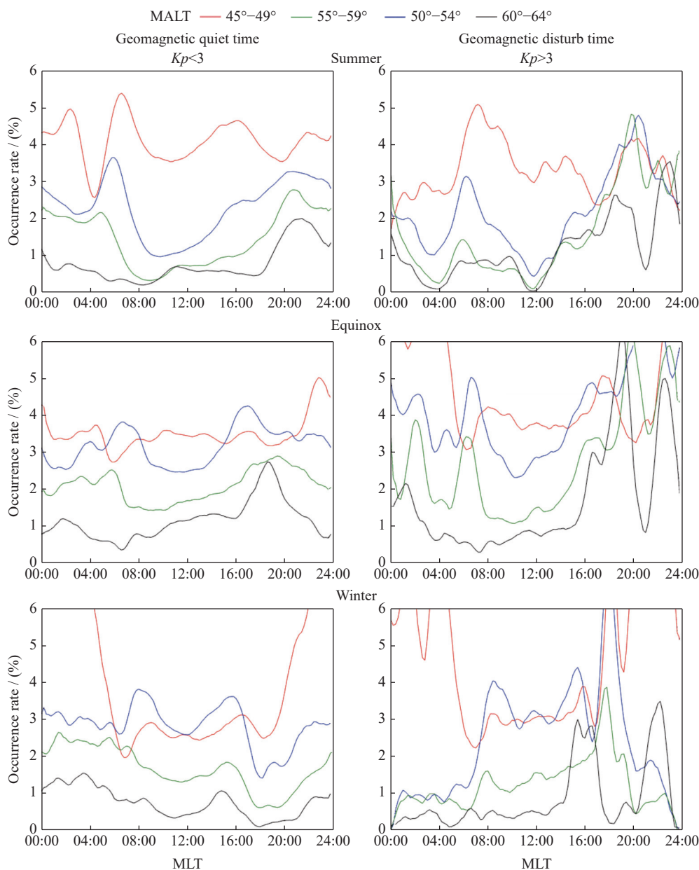
图 5 不同季节与不同地磁条件下 HOK 雷达观测到的不同纬度范围回波发生率随时间的变化
