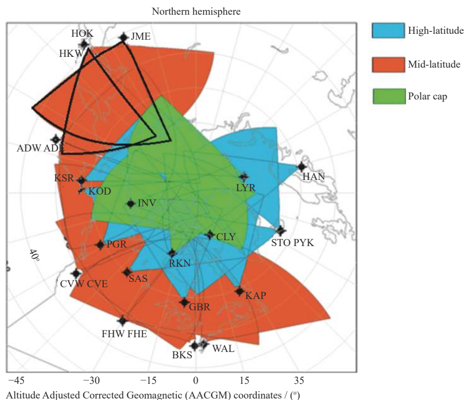
图 1 北半球 SuperDARN 雷达视野 (粗黑线标出部分为 JME 雷达和 HOK 雷达视场)
