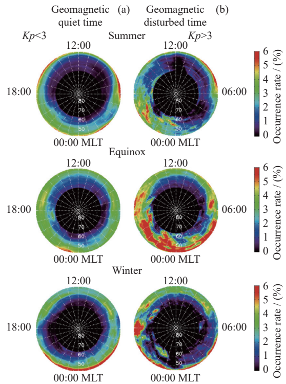
图 3 2018 年 3 月至 2019 年 11 月不同季节 HOK 雷达在地磁平静期和扰动期的回波发生率分布
