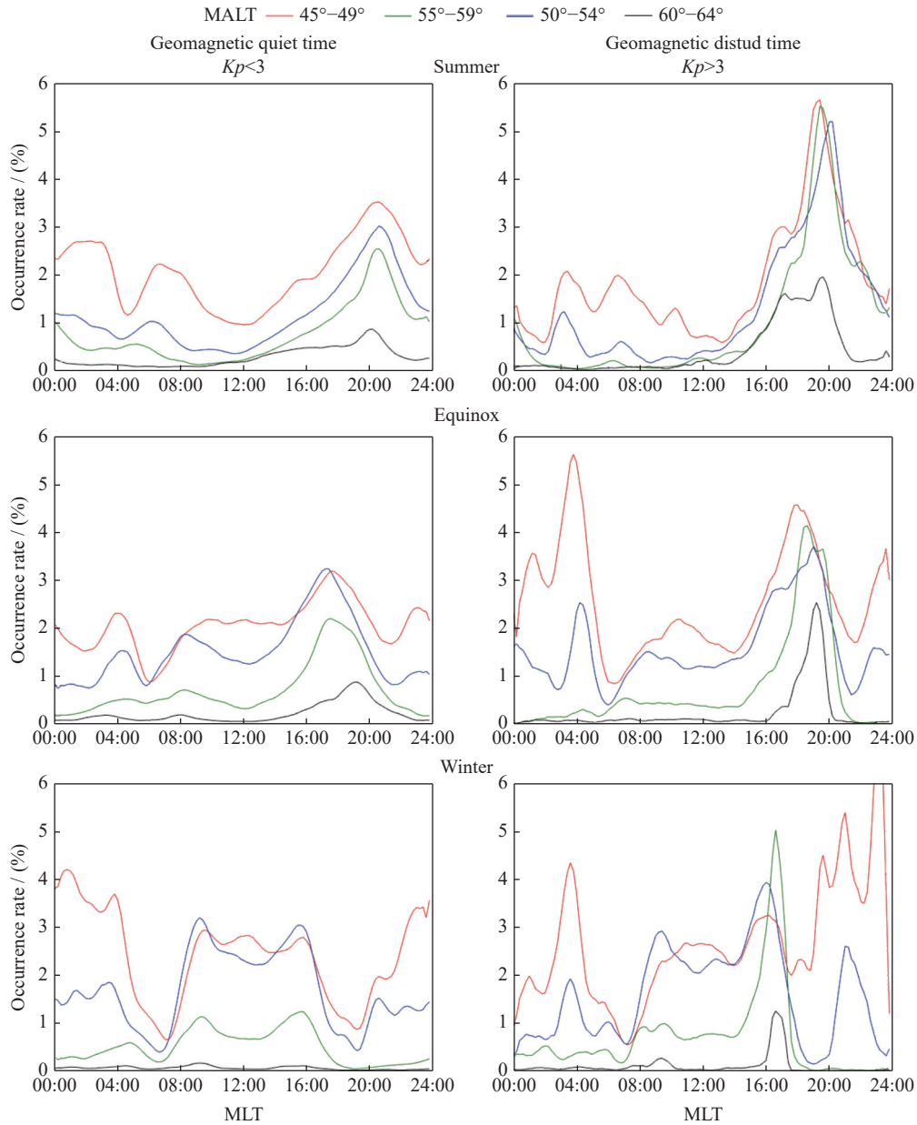
图 4 不同季节与不同地磁条件下 JME 雷达观测到的不同纬度范围回波发生率随时间的变化
